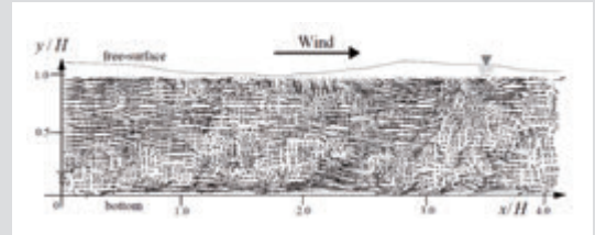
モデル実験で捉えた沿岸吹送流の乱流構造
