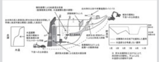
ダム貯水池の環境影響緩和策
