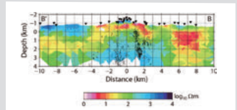
箱根火山の地下比抵抗構造
