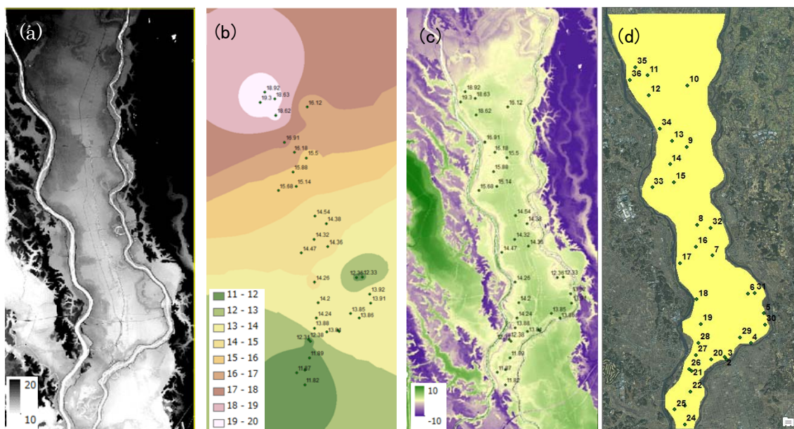
図1 浸水深分布の推定手順：(a) 5m 空間分解能の数値標高モデル、(b) 35 地点の計測浸水位とその空間内挿、(c) 浸水位－標高（単位はいずれも[m]）、(d) 本解析の対象領域マスク
