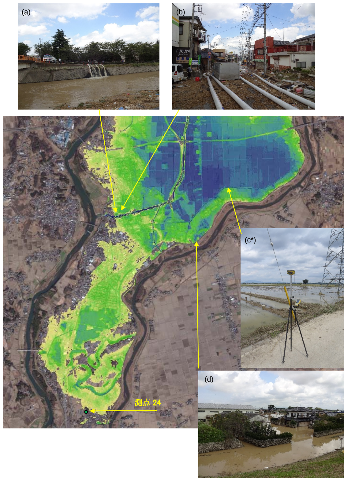
図3 最大浸水深分布の推定結果（南部：水海道周辺）（凡例は図2と同じ）
