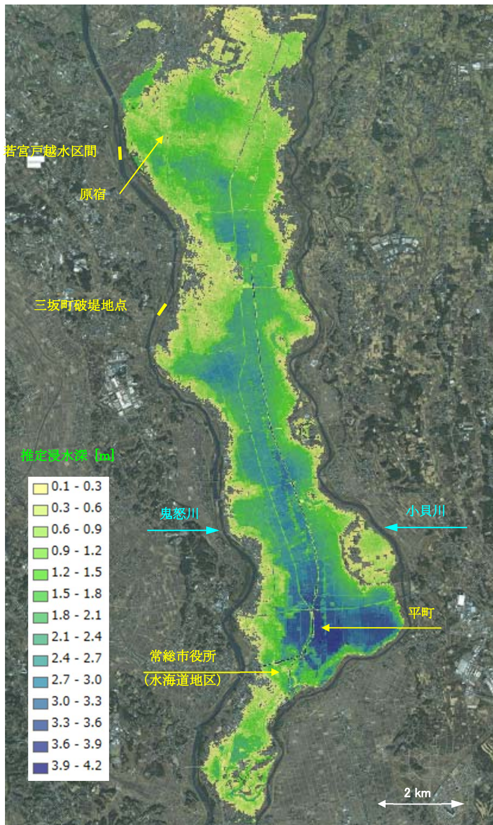
図2 最大浸水深分布の推定結果
