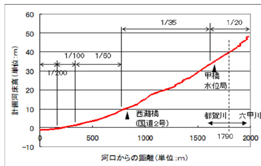
縦断面図
