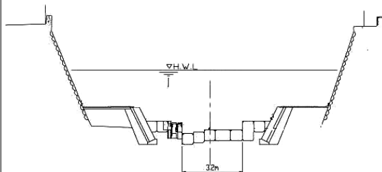
横断面図 (西灘橋付近(国道2号))
