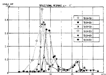
Fig. 16. Velocity-Amplitude Curve.
