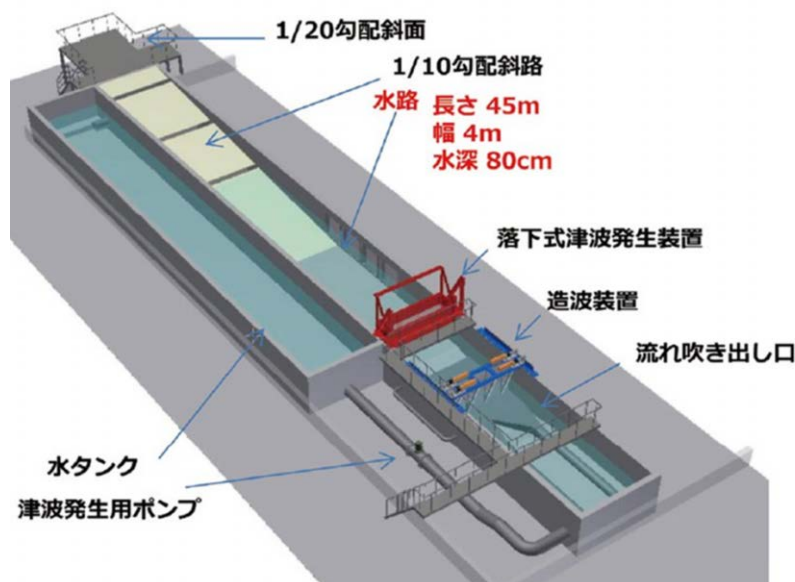
津波再現水槽の外観図
