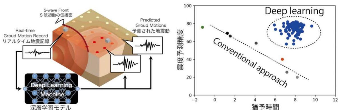
図2 機械学習によるリアルタイム地震動予測の概念と緊急地震速報への適用事例
