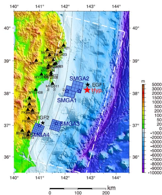
平成23年東北地方太平洋沖地震の強震動生成域
