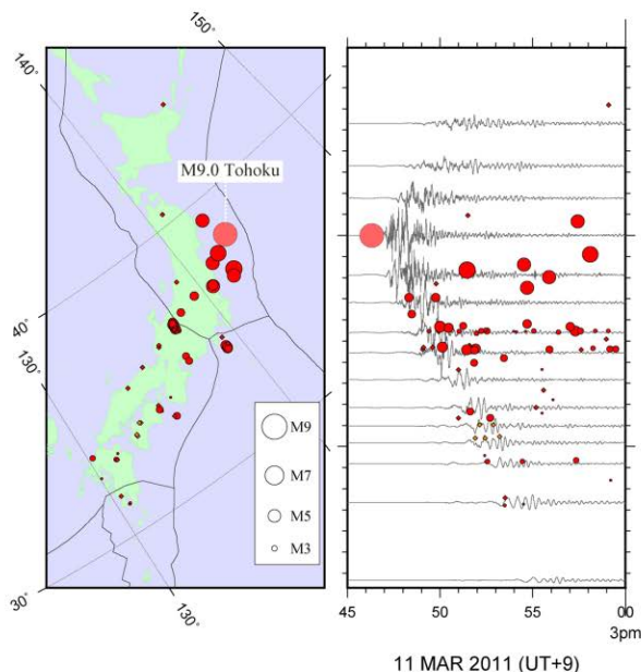
平成23年東北地方太平洋沖地震による動的誘発地震の検出
