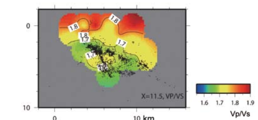
長野県西部地震の震源域における地震波速度構造（Vp/Vs比）と地震分布の関係。Vp/Vs比の小さなところで地震が発生している。Relationship between Vp/Vs ratio and hypocentral distribution in the Western Nagano prefecture region. Microearthquakes are concentrated in the region with low Vp/Vs ratio.
