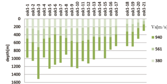
大阪平野南部における常時微動の水平上下スペクトルから同定した地下構造モデル Subsurface structure of the southern part of Osaka plain identified from Horizontal-to-Vertical spectral ratio of microtremors
