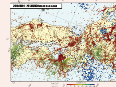
西南日本の地震活動（2010年1月～2013年6月） 大学の観測網等のデータも利用して気象庁が決定した震源カタログによる。最新の震源分布はセンターのWebサイトでご覧いただけます。
