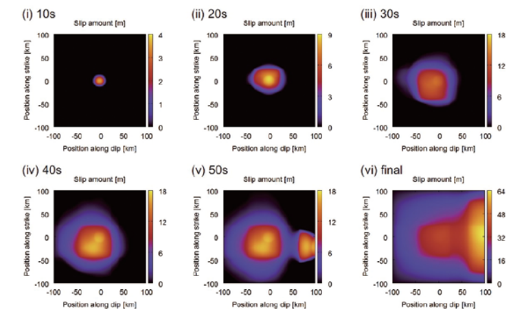
東北地方太平洋沖地震の動的破壊シミュレーション（TPを考慮） Dynamic rupture simulation for the 2011 Tohoku Earthquake considering the effect of thermal pressurization
