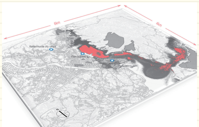
図2 2011年東北地方太平洋沖地震で発生した津波による気仙沼湾の石油流出火災の再現シミュレーション
